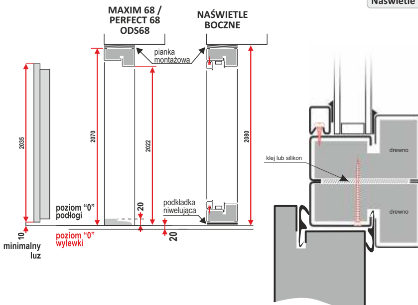
ŁĄCZENIE NAŚWIETLA Z OŚCIEŻNICĄ - GÓRNY RÓG
